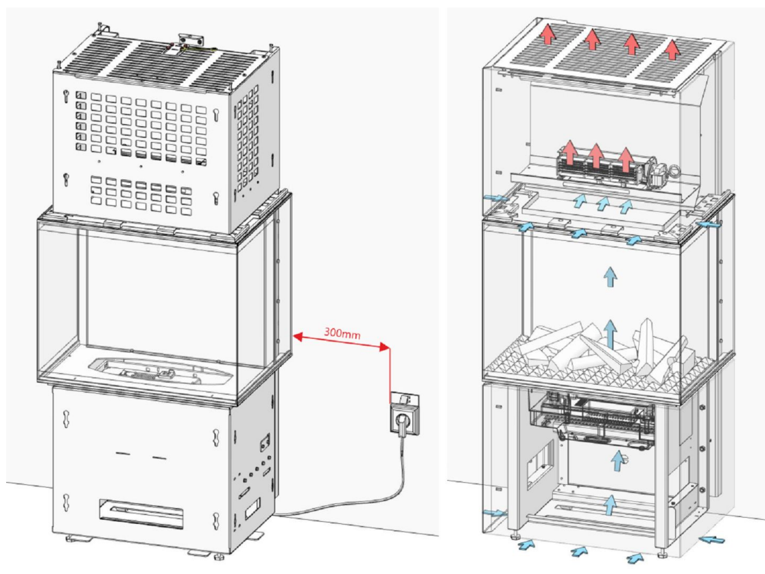
Rys. 1 Przykład instalacji urządzenia i przepływu powietrza
