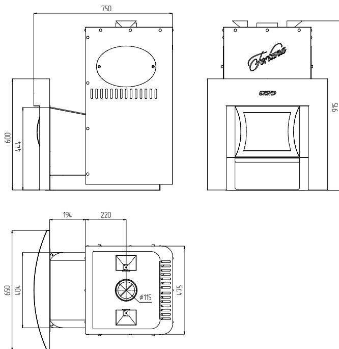
Рис. 1 Размерные характеристики печи «Grill'D» Fortuna 200 window
