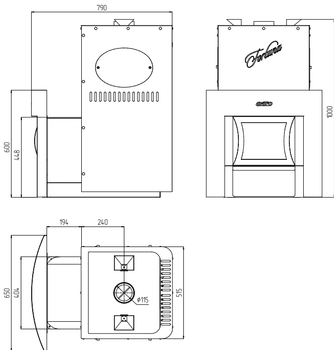
Рис. 1 Размерные характеристики печи «Grill'D» Fortuna 280 window
